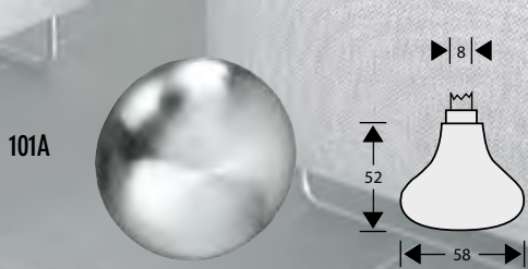
PADDESTOELMODEL ROND 58 MM. GATDEEL KLIKAANSLUITING.
