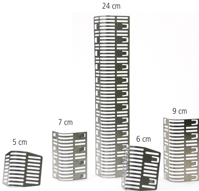
Standaard hoogtematen: 5cm - 6cm - 7cm - 9cm - 24cm
