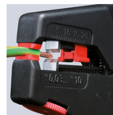
12 40 200: Precies afstrippen zonder de ader te beschadigen
