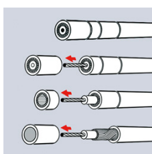
Driedelig afstrippen van een coax-kabel
