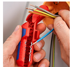
Afstrippen van individuele geleiders
