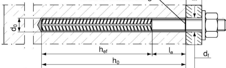
fischer rebar anchor FRA Pre-positioned anchor
