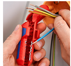
Dénudage de conducteurs individuels
