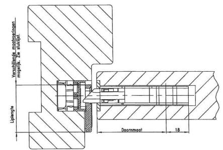
Doorsnede deur en kozijn
