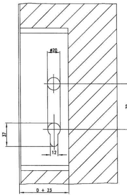
Frezing voor de Hoofdslotkast
