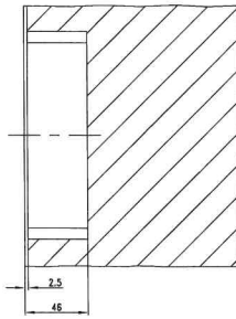
Frezing voor bijzet slotkast voor automatic schoot
