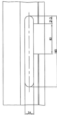
Frezing in kozijn voor sluitkom hoofdslot
