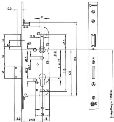
Maatvoering hoofdslotkast
