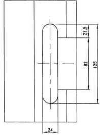
Frezing in het kozijn voor sluitkom automatic
